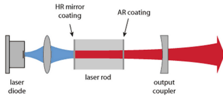
Obr. 2: Podélné diodové čerpání [4]
