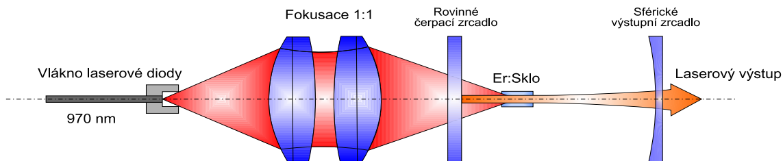
Zjednodušené schéma laserového rezonátoru s aktivním prostředím
